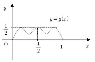
[그림7] g(x) = f(\sin^2 \pi x) 그래프 (EBS)
